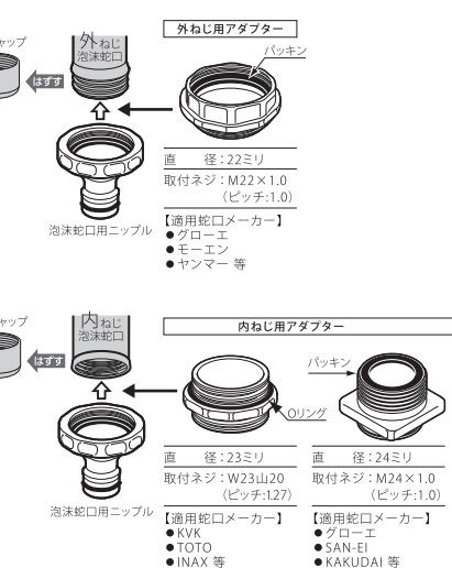
G063 泡沫蛇口用ニップル
