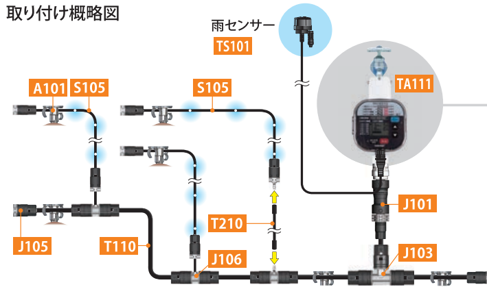
かんたん水やりタイマー
