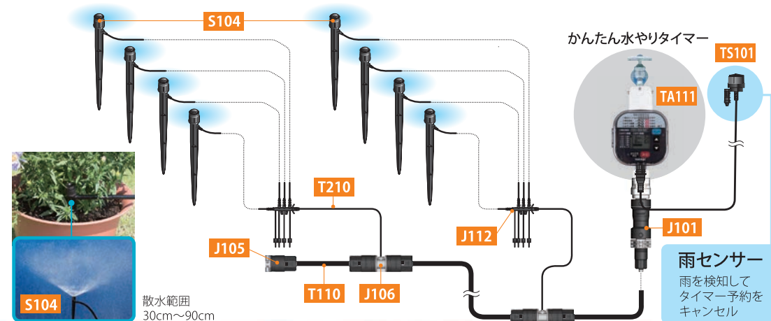
取り付け概略図
